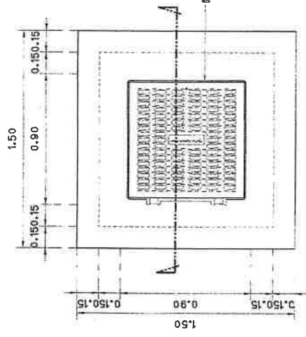
แบบขยายบ่อพัก(หัวมุม) มาตราส่วน 1 : 25
