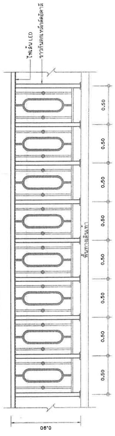
รูปด้านติดตั้งราวกันตกเหล็กดัดอีตาดี
